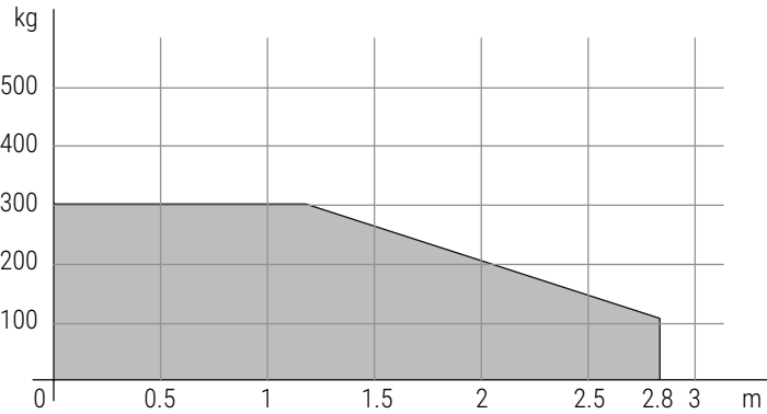
BE20/200
