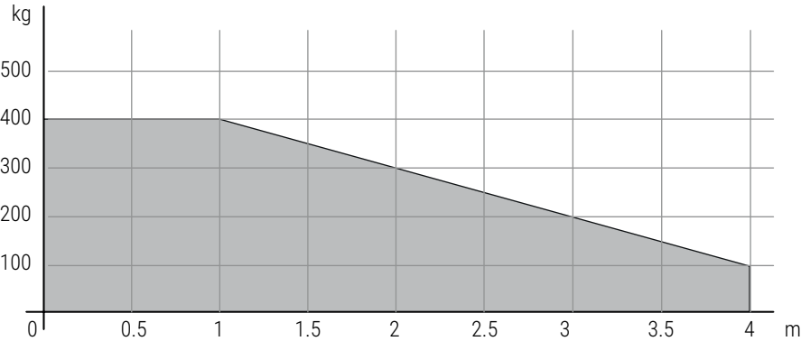
BE20/400
